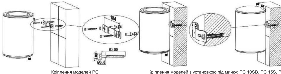
Рисунок 4. Кріплення ЕВАД до стіни
