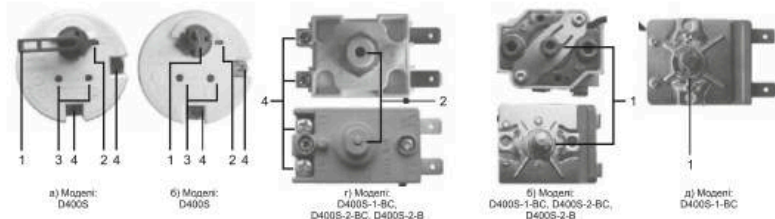
Рисунок 3. Зовнішній вигляд терморегулятора
