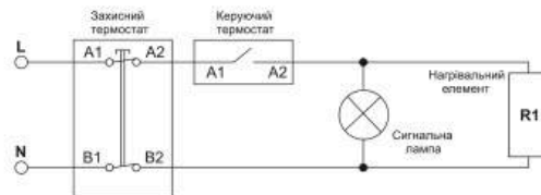
Рисунок 7. Схема електрична для моделей: D400S-1-BC, D400S-2-BC, D400S-2-B
