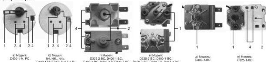
1 – Регулятор температури; 2 – Кнопка теплового захисту; 3 – Місце підключення сигнальної лампи; 4 – Клемні колодки для підключення до електромережі
