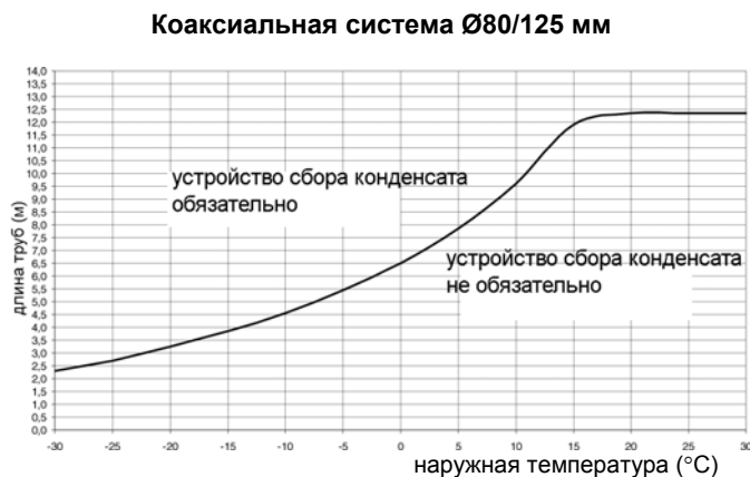
Коаксиальные дымоотвод/воздуховод
