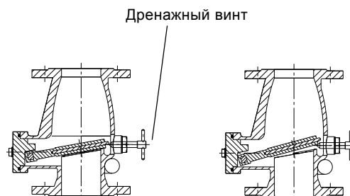
Рис. 20 Дренажный винт для обратного клапана multilift MLD
