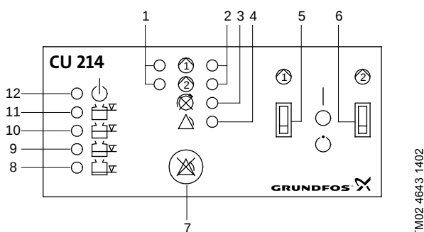
Рис. 24 Пульт управления модуля CU 214
