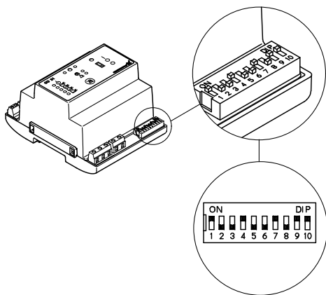
Рис. 22 Модуль CU 211 с микропереключателем
