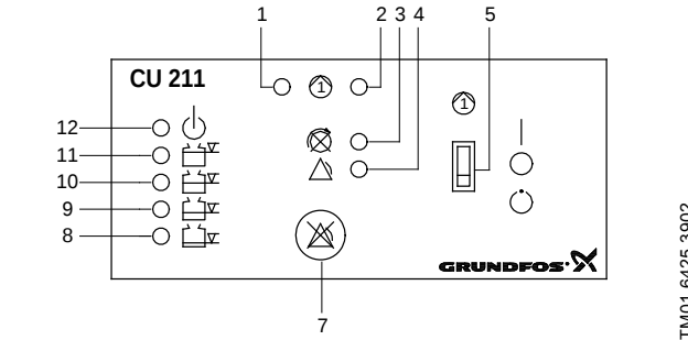
Рис. 21 Пульт управления модуля CU 211
