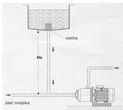
Рис. 5 Слив жидкости
