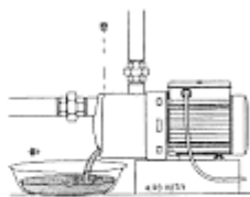
Рис. 5 Слив жидкости
